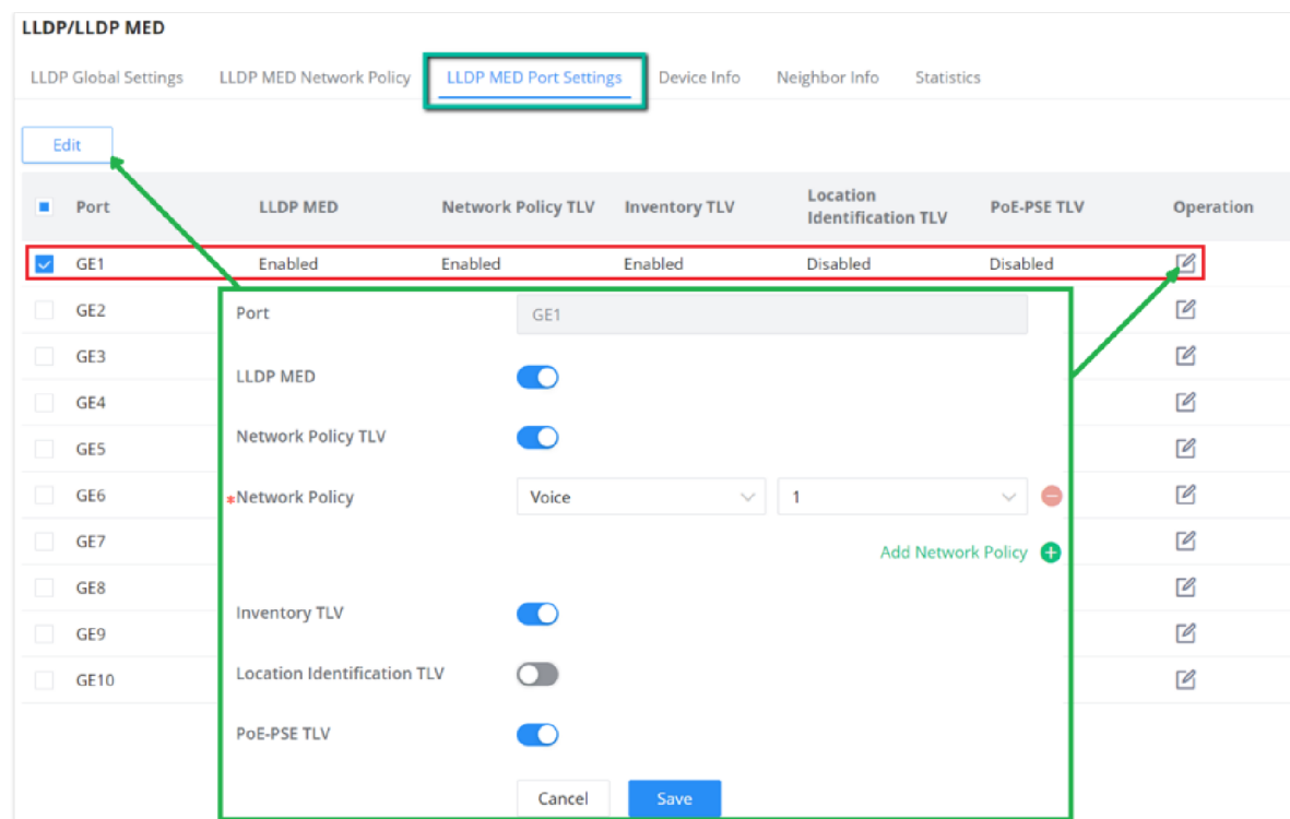
LLDP MED Port Settings
